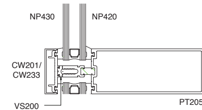
② JAMB
